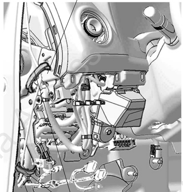
车辆线束 线束胶带(2)
